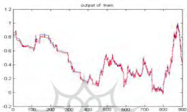
نمودار ۴. نمایش خروجی شبکه (به رنگ قرمز) به همراه خروجی مطلوب (به رنگ آبی) با استفاده از داده آموزش
