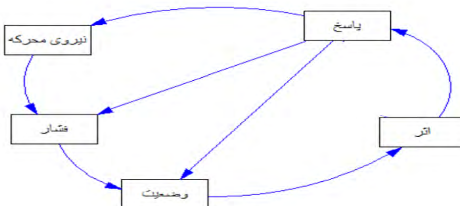
شکل ۱. مدل DPSIR
