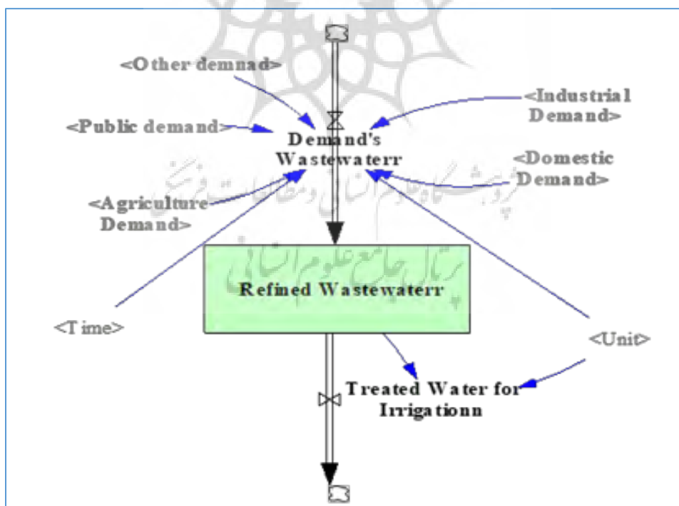
شکل ۳- نمودار حالت و جریان زیر سیستم تصفیه فاضلاب
