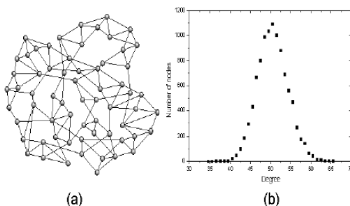
شکل ۵- گراف حاصل از مدل جهان کوچک، (a) مدل جهان کوچک، (b) توزیع درجات ۱۰ گراف با ۱۰۰۰ گره و p=0.3 (هلمی، ۲۰۱۸)
