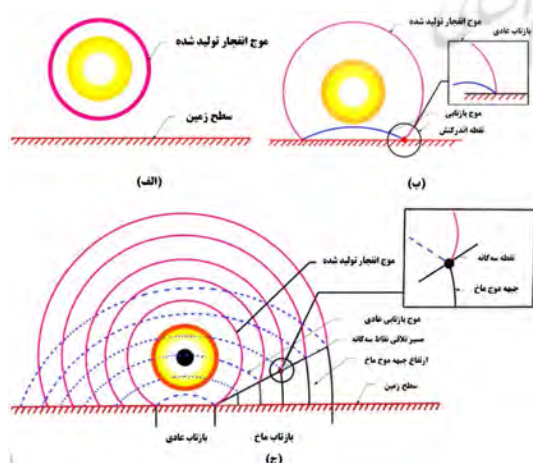
شکل ۱. مکانیزم تولید جبهه موج ماخ (Shirbhate & Goel, 2020)
